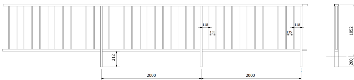
Módulo estándar
